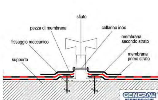
Fig. 22 - Sfiato/Areatore con fissaggio meccanico
