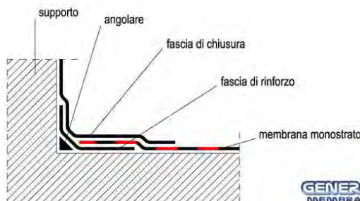
Fig. 15- risvolto verticale: posa in monostrato senza fissaggio meccanico
