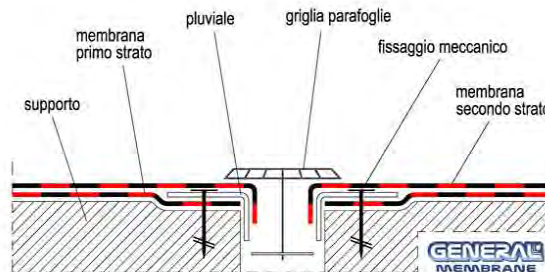
Fig. 14 – Scarico di un Pluviale
