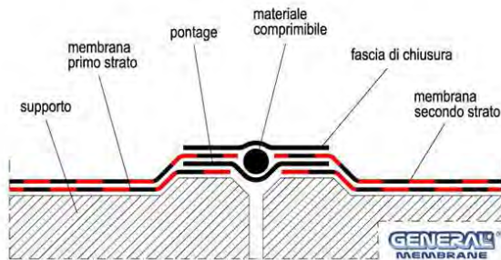
Fig. 30 – Giunto di dilatazione piatto – tetto freddo
