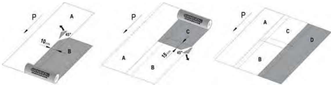
Fig.9 – posa in MONOSTRATO o PRIMO STRATO: posizionamento teli e esecuzione saldature sezione corrente (le lettere indicano la successione di posa dei fogli con indicazione delle misure delle sovrapposizioni laterali e di testa)
