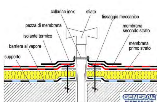
Fig. 25 - Sfiato doppio corpo collegato a ambienti interni
