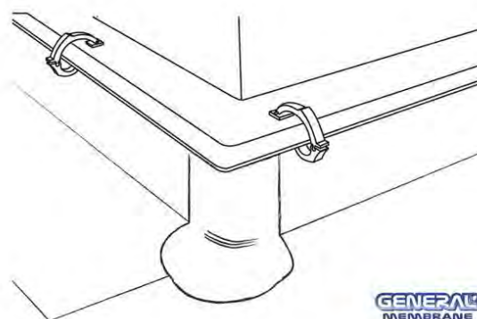
Fig. 29 – lucernaio: rinforzo dell’angolo
