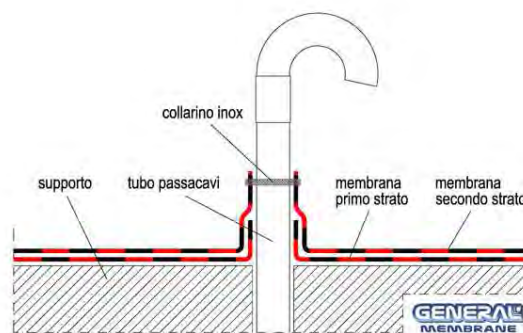
Fig. 27 – Tubo passante senza pezzo speciale
