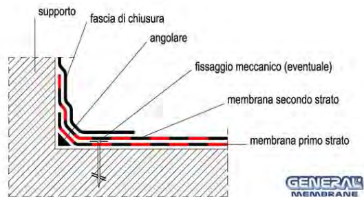
Fig. 18 - risvolto verticale doppio strato – Tipo 2
