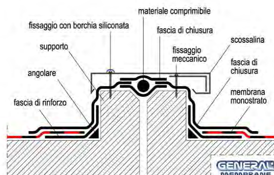
Fig. 32 – Giunto di dilatazione in rilievo
