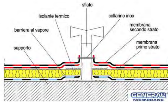
Fig. 23 - Sfiato su estradosso con stratigrafia coibentata
