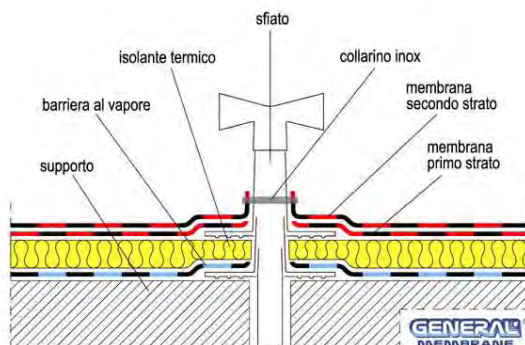
Fig. 24 - Sfiato doppio corpo collegato alla barriera al vapore
